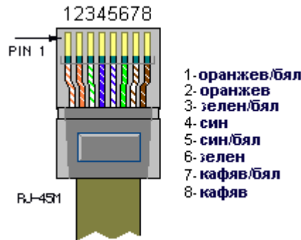
Фигура 2: Схема на конектор RJ45
